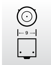
Bay9s
