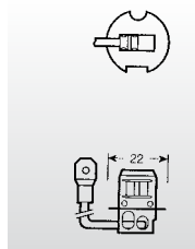
PK22s
