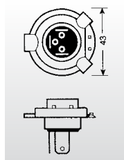
Px43t
