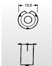
P13,5s
