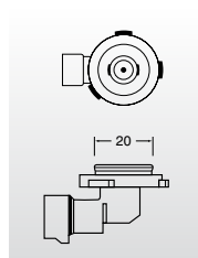
Pz20d
