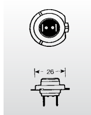
Px26d
