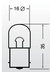
tubular
