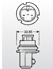
P29t
