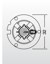
D2R
