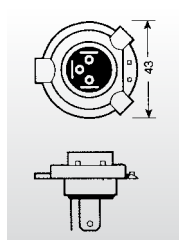
Px43t
